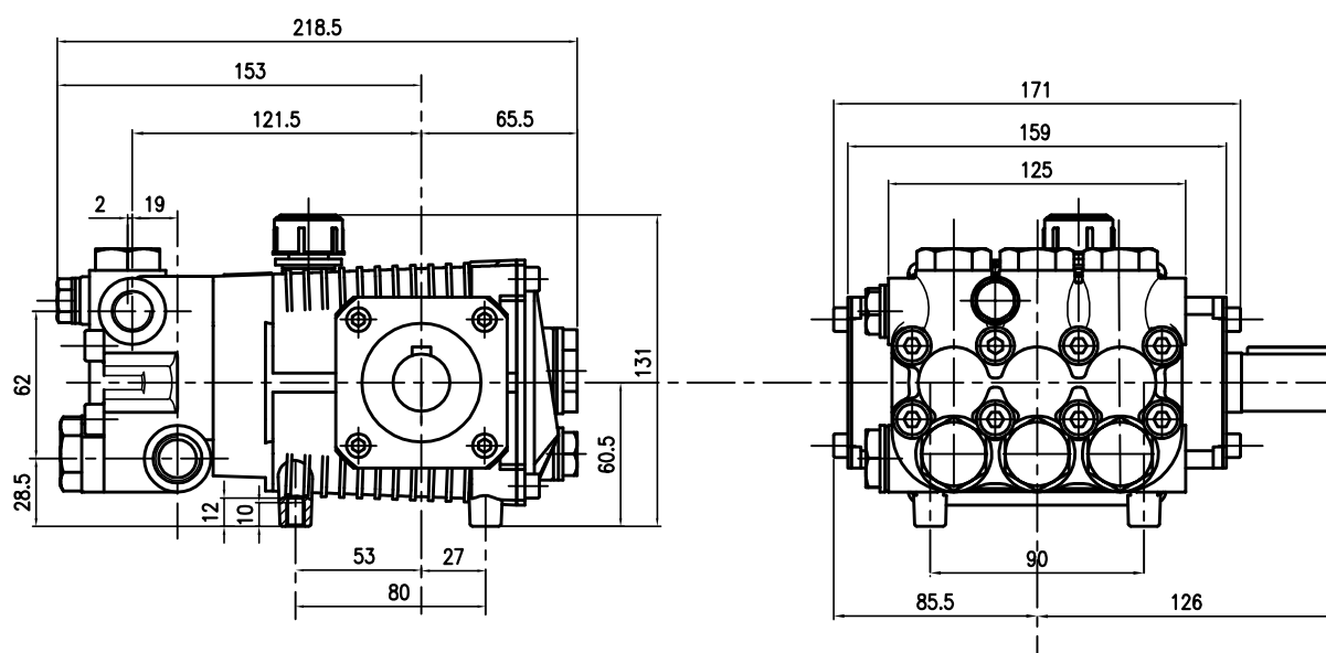
HD8515-HD1015-HD1115-HD1215-HD1315-HD1415
